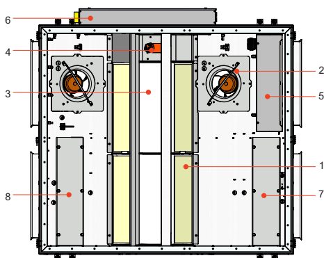
Рис. 6.1. RIS 1200 P EKO 3.0
