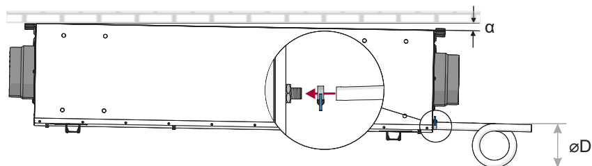
Рис. 13.1.2. установка дренажа ( \phi D = 150 mm)
