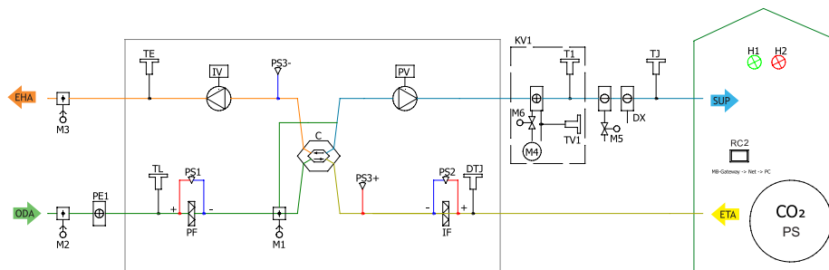
Рис. 15.1. RIS PE EKO 3.0
