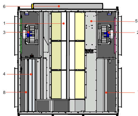
Рис. 6.2. RIS 1900-2500 P EKO 3.0
